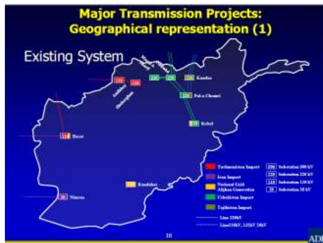
شکل 1: مسیر های عمده لین های انتقال برق [1].
